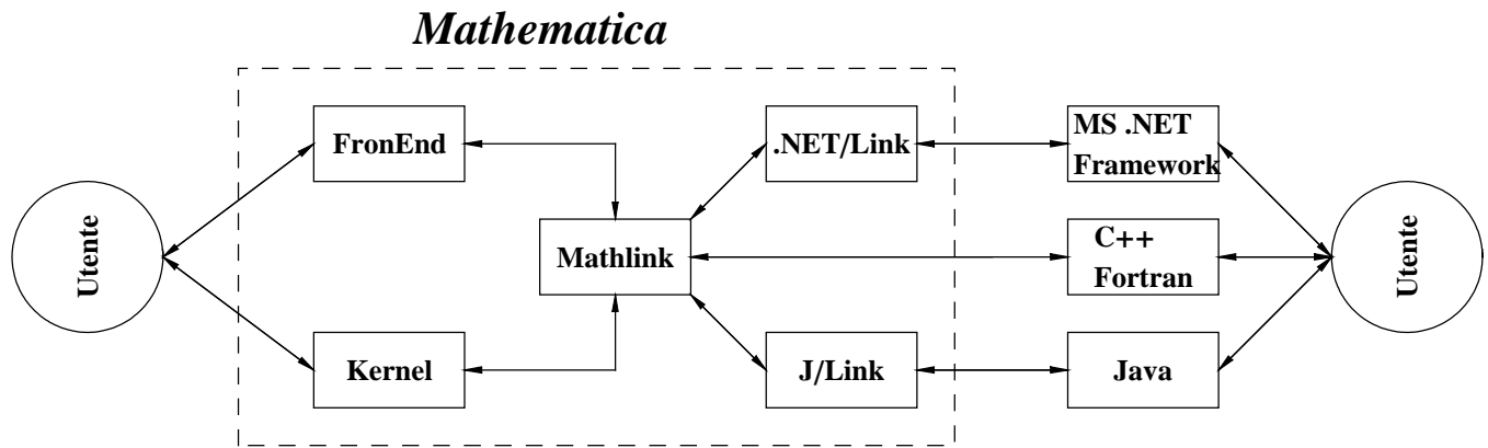
Figura 1. Architettura interna di Mathematica .
